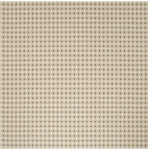
Nougat
